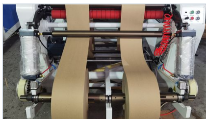
选配 双卷放料套件 OPTIONAL · DUAL-ROLL UNWINDING
